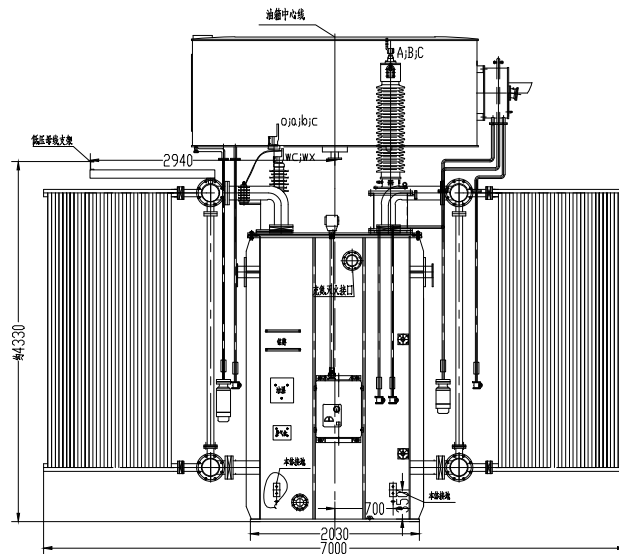
本体及铁心附件接驳示意图
