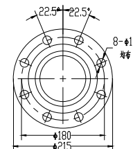
100侧门法兰(注油油)尺寸
