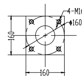
80抽气孔罐网法兰尺寸
