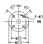
25侧门法兰尺寸
